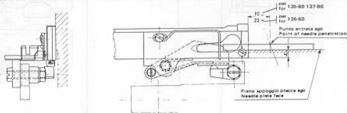
SCHEMA DI MONTAGGIO APPAR. 135-80; 136-80; 137-80 CON AZIONATORE A LEVA PER MACCHINE SENZA TRASPORTO DIFFERENZIALE LAYOUT FOR MOUNTING THE 135-80; 136-80 137-80 DEVICES WITH LEVER STARTER FOR HEADS WITHOUT DIFFERENTIAL FEED
