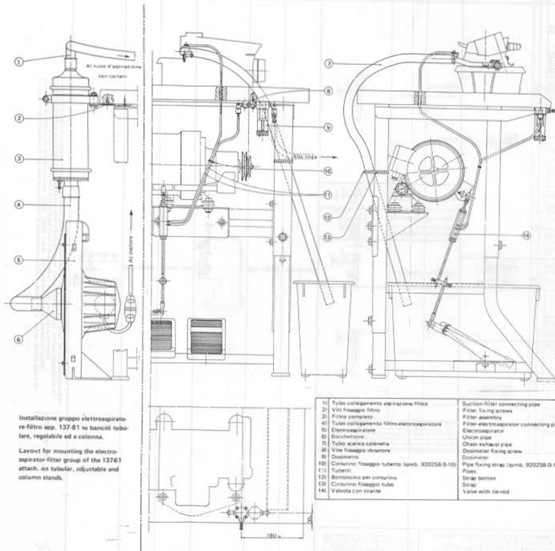
Installazione app. 135-81 e 136-81 su bancali tubolare e regolabile Layout for mounting the 135-81 and 136-81 att. on tubular and adjustable stands.
